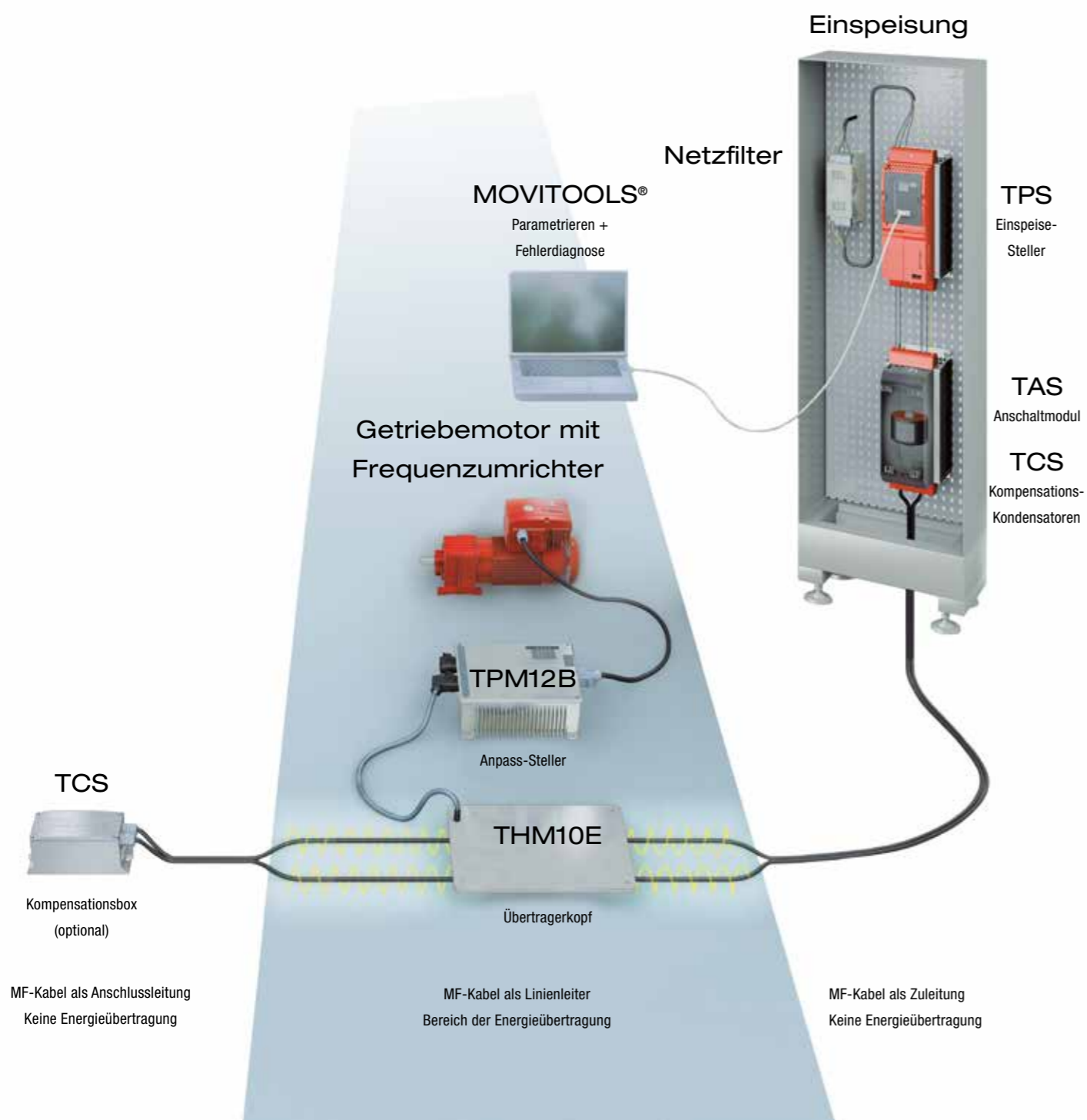
MOVITRANS® mit flachem Übertragerkopf (THM10E)
